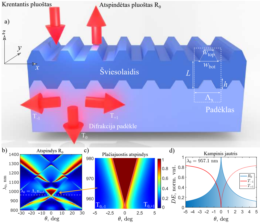
6.8 pav. Trapecijos formos šviesolaidinis filtras (a), filtruojantis kritusią šviesą per difrakciją, o filtruotas pluoštas yra atspindėtas. Šios struktūros atspindžio skirstinys iliustruojamas (b) grafike, kuriame matyti plačiajuostis atspindys (priartintas, c). Jo difrakciniai efektyvumai nurodyti (c) grafike, kur raudonos kreivės atitinka \pm 1 difrakcinės eilės.
