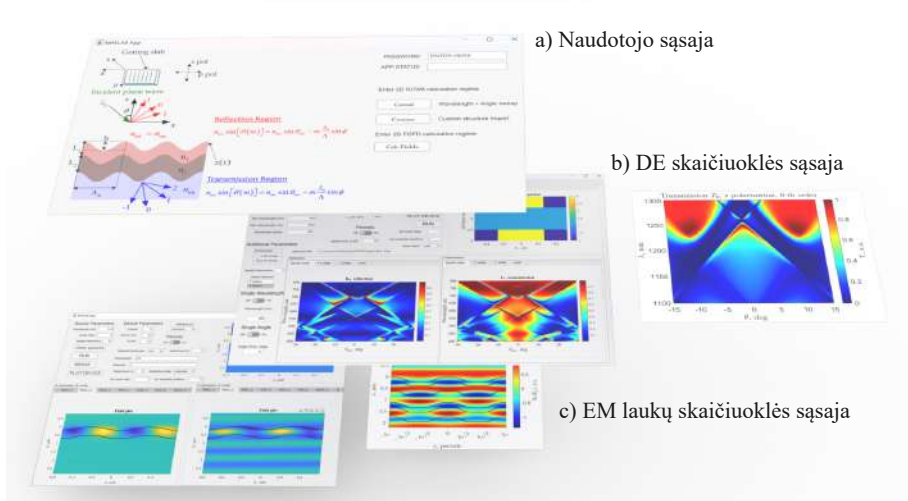
6.12 pav. Vartotojo sąsaja "ZenScat" su atidarymo programėle a), difrakcinių efektyvumų skaičiuokle b) ir EM laukų skirstinių skaičiuoklės sąsaja c).
