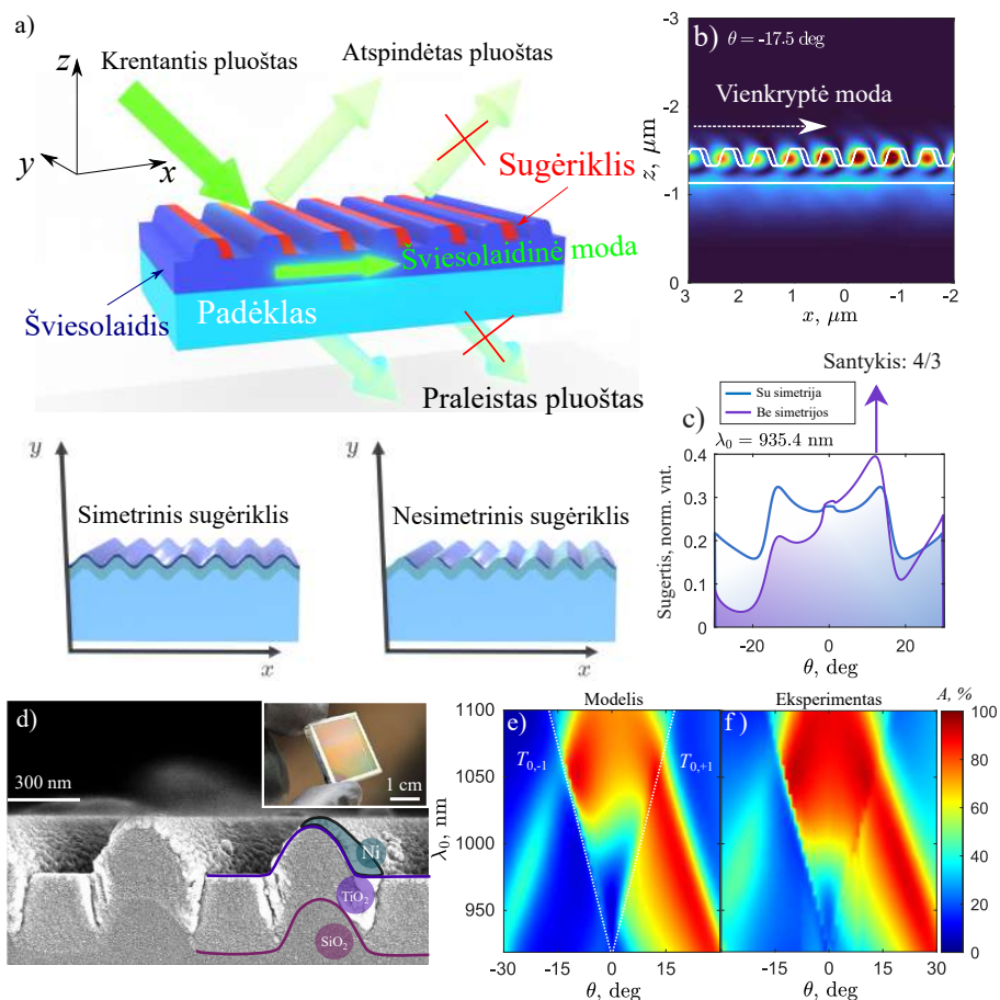
6.10 pav. Viena kryptimi sklindančios šviesolaidinės modos koncepcija (a ir b), kur dėl nesimetriškai išdėstyto sugėriklio padidėja sugertis (c). Dviguba moduliacija pasižymintis supergausinis filtras (d) ir jo atitinkamai paskaičiuoti (e) ir išmatuoti (f) sugerties spektrai.
