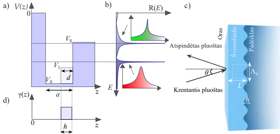
6.9 pav. Potencinės duobės schema (a) su surištų būsenų rezonansais (b). Ši schema atitinka šviesolaidinių modų filtro struktūrą (c). Moduliacijos gylis h atitinka sietį tarp kritusio šviesos pluošto, šviesolaidinės modos ir atspindėto lazerio pluošto, kuris pavaizduotas d).
