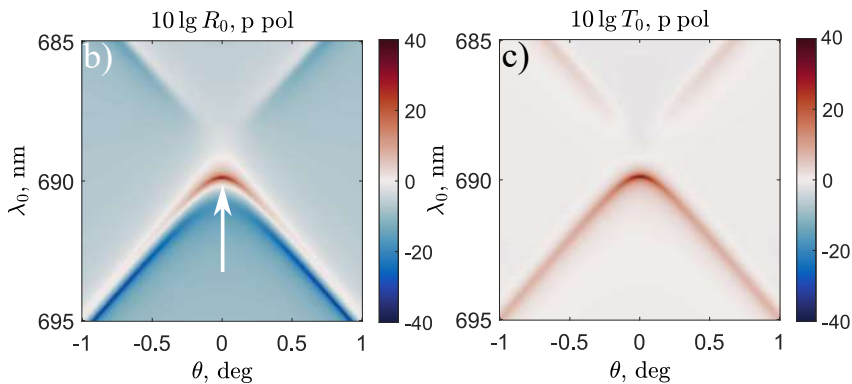
6.11 pav. Aktyvios šviesolaidinės terpės su harmonine moduliacija dizainas (a) bei atspindžio (b) ir pralaidumo (c) spektrai p poliarizacijai.
